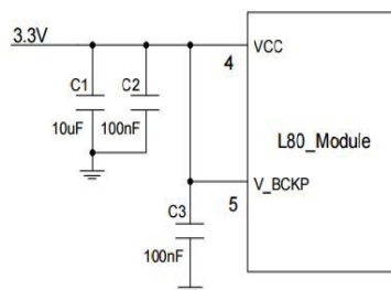
Figura 1: Esquema de referencia del circuito de potencia
